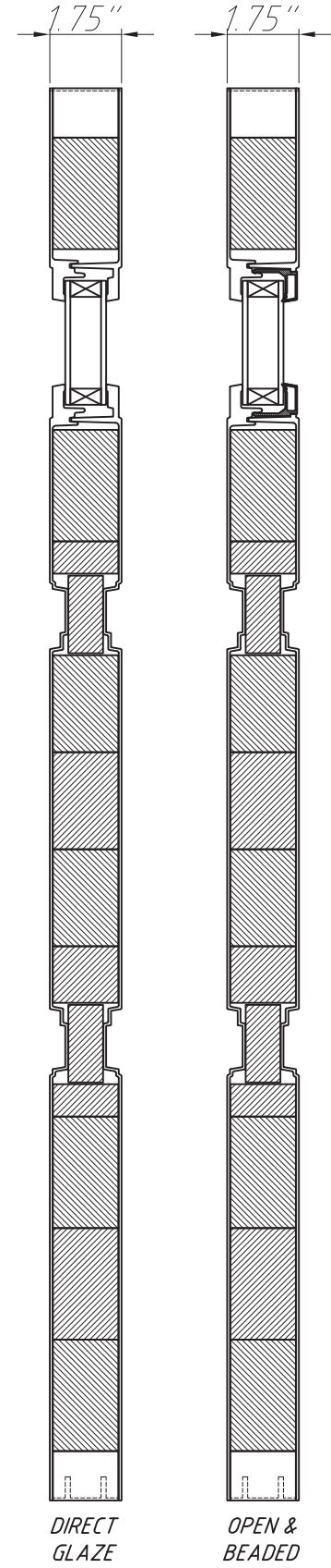
Section A-A
