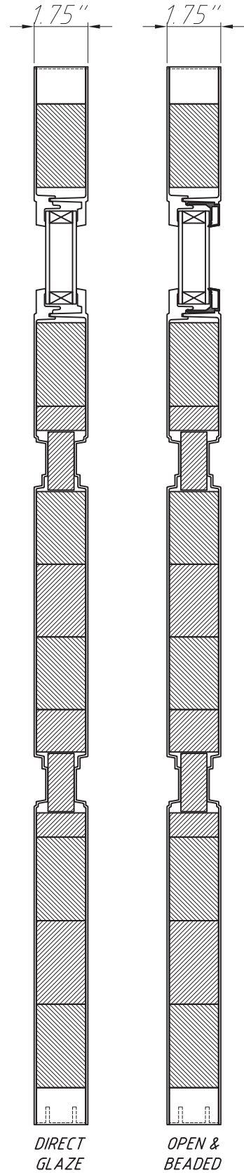
Section A-A
