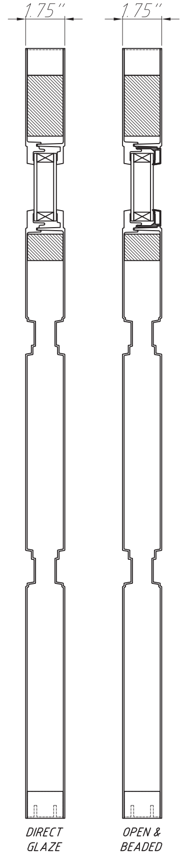
Section A-A
